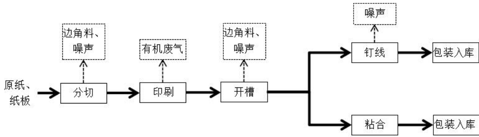
图 2-3 纸箱生产工艺及产污环节图
