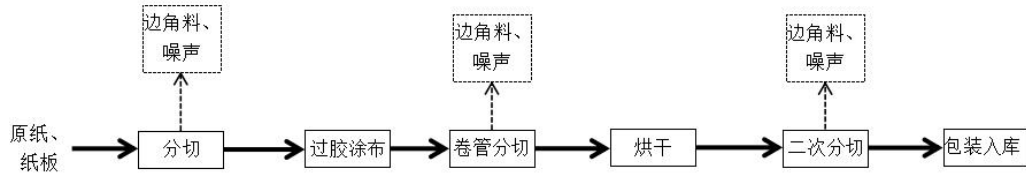
图 2-2 纸管生产工艺及产污环节图
