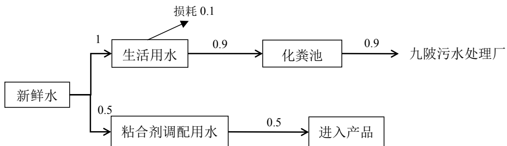
图 2-1 本项目水平衡图（单位： \text{m}^3/\text{d} ）
